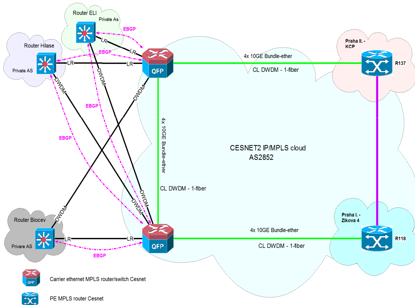
Návrh logické topologie připojení ELI, Hilase a Biocev
